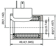
DIN 4365/A-ISO 4400
