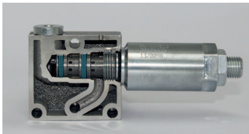
Een voorbeeld van een direct bediend ventiel, geoptimaliseerd voor 3D-printen. Deze ventielen worden getest tot 350 bar wat ze moeiteloos doorstaan.
